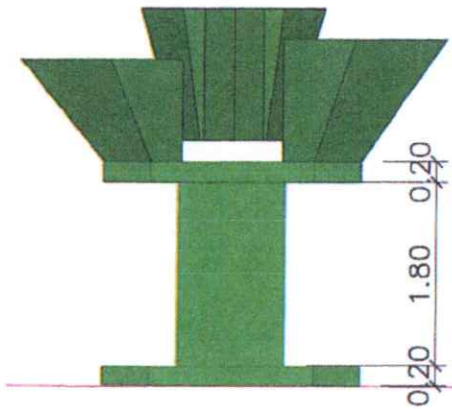
FRONT VIEW SCALE N.T.S.
