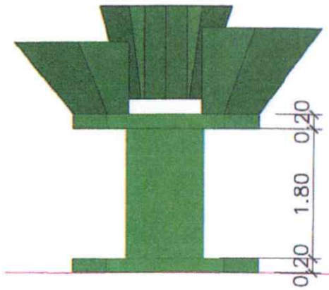
FRONT VIEW SCALE N.T.S.
